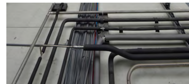
RVS leidingwerk
